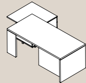
Scrivania con mobile di servizio integrato decentrato / Desk with integrated service element decentralized L 235 P 135 H 75
